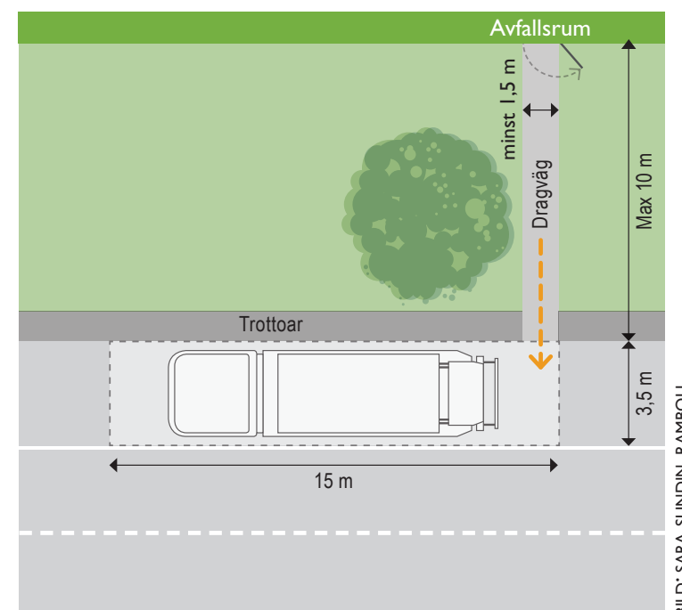
Figur 2: Utformning dragväg
